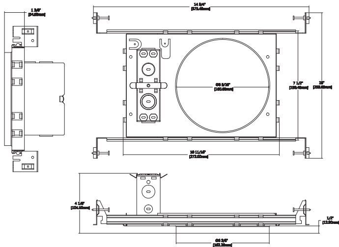
DLFRAME/C6R
